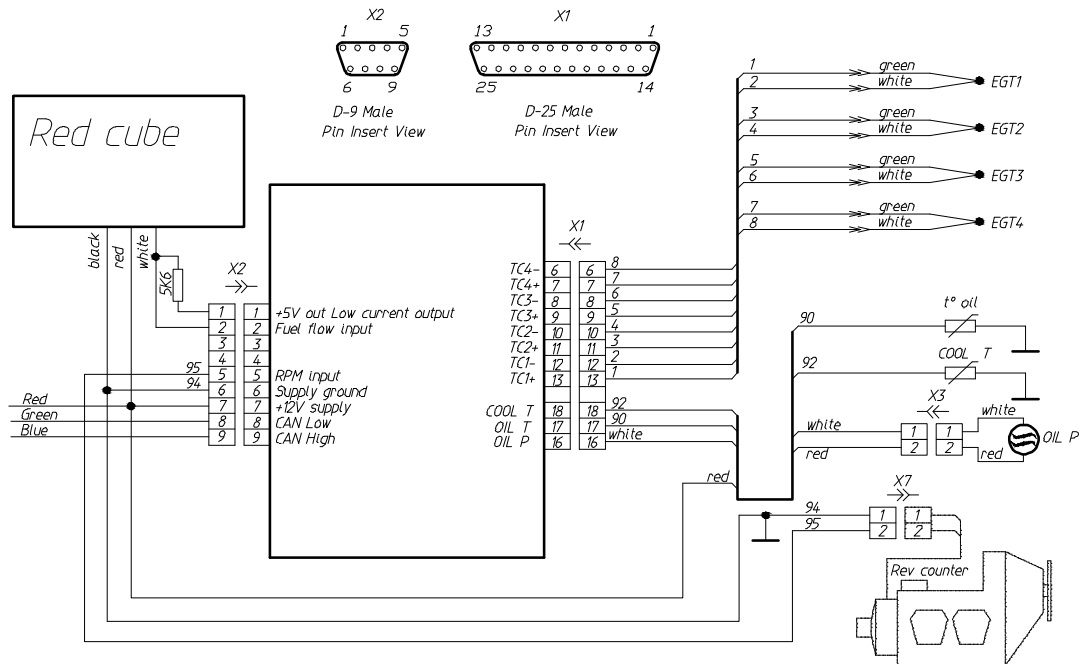
Kabelbaum MGL RDAC XG
