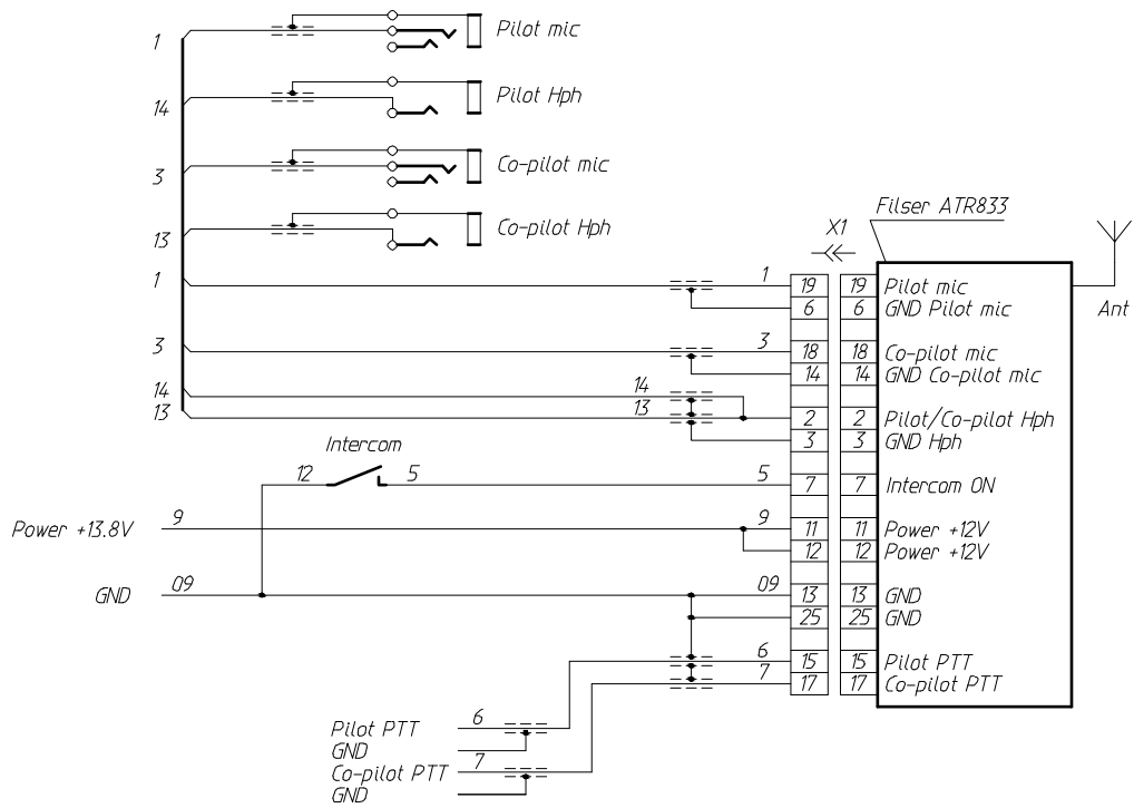
Kabelbaum Rundfunk FUNKE ATR833
