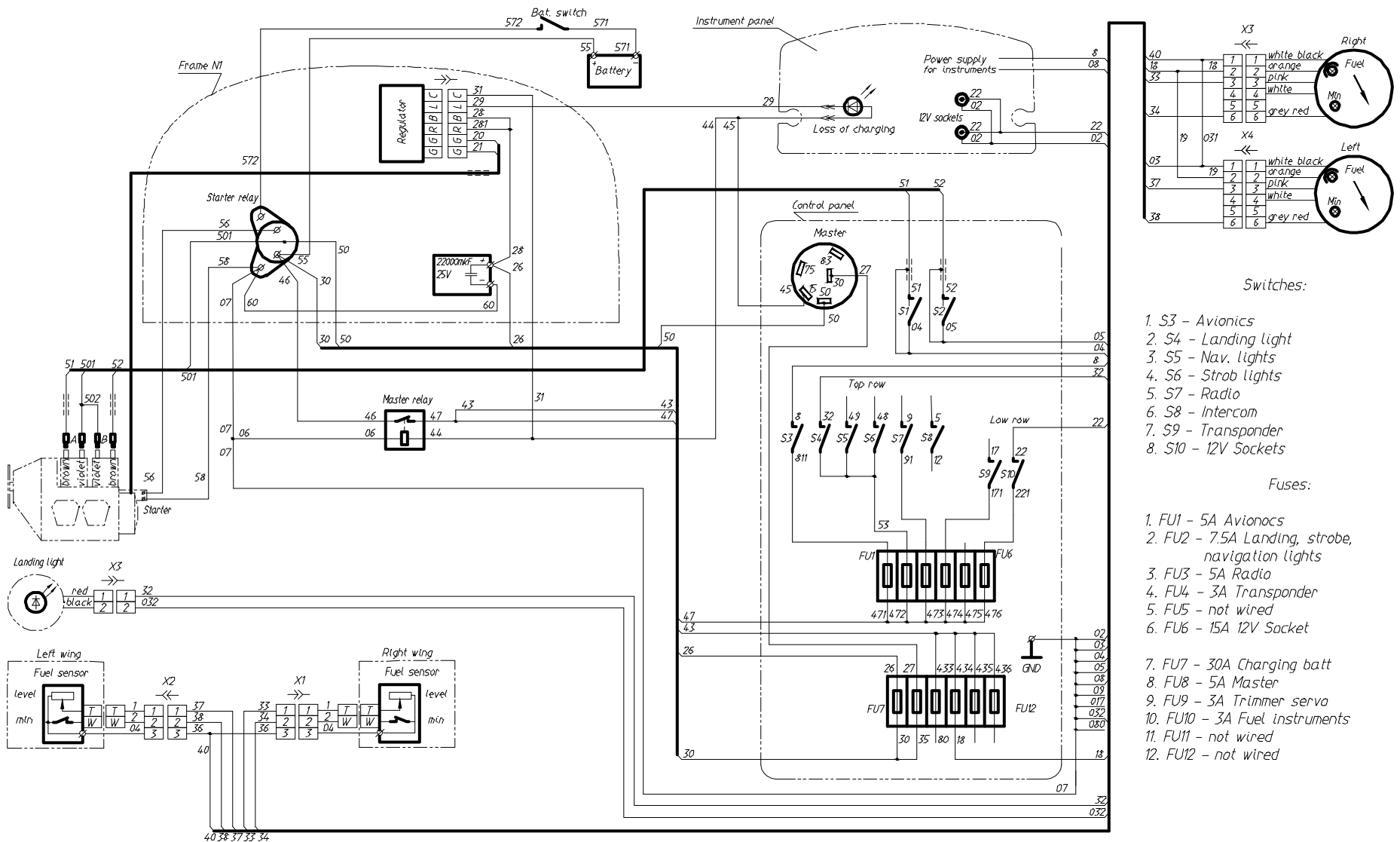
Elektrische Anlage A-22L2 Seriennummer 525
