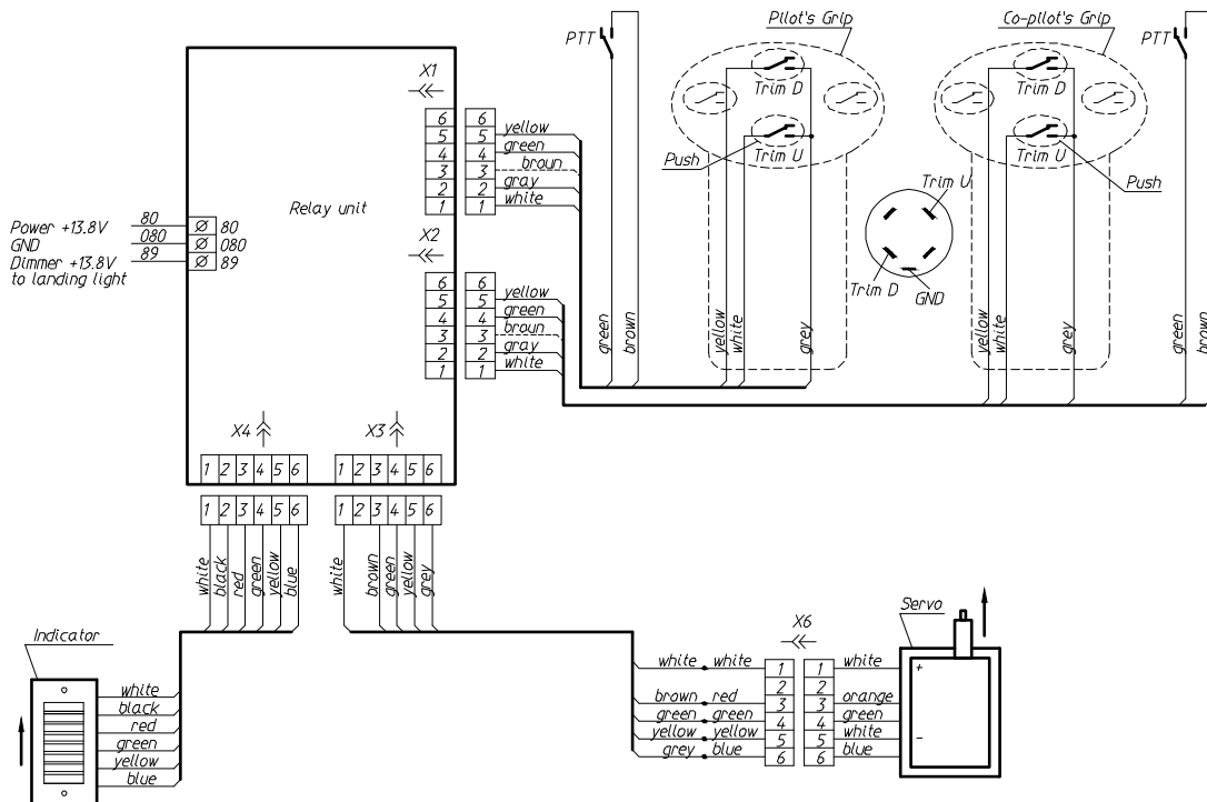
Kabelbaum elektrische Trimmung
